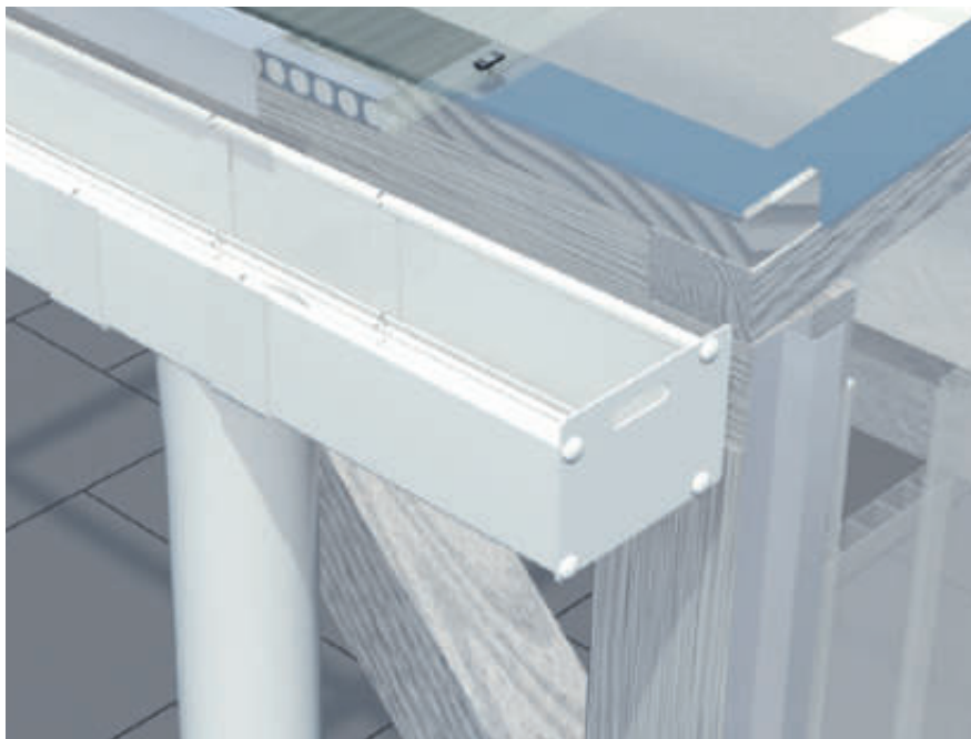
7 Dachrinnen Für die zuverlässige Entwässerung hochwertiger Überdachungen bis 51 qm Grundfläche. Die runde owolux® aus Hart-PVC oder die eckige alwo® aus Aluminium. Beide überzeugend in Qualität und Funktion. Die owolux® Dachrinne ist für freie Spannweiten bis max. 600 mm von Sparren zu Sparren geeignet. Für größere Spannweiten sollte die alwo® Dachrinne genutzt werden, hier sind Spannweiten bis 1.250 mm möglich.
