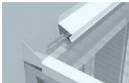
5 Wandanschlussprofil Mit zusätzlichen Seitenblenden ist der Anschluss zur Hauswand gesichert. Die Fuge ist mit Plexisil abzudichten.
