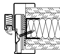
Diagonalfestigung (Porenbeton)
